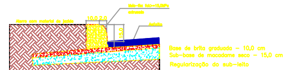
Detalhe do meio fio – trecho sem calçamento
