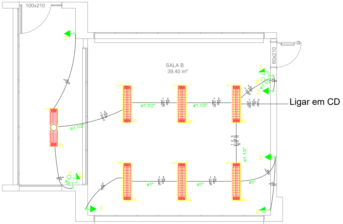
Detalhe Elétrico Sala B
