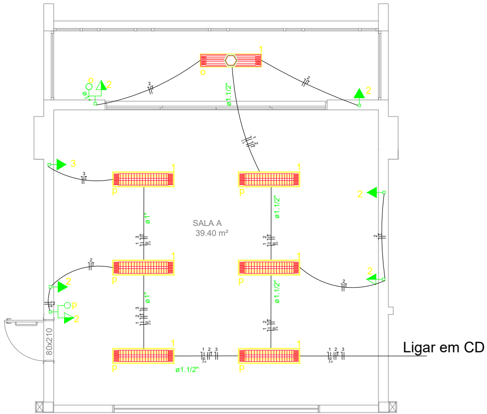
Detalhe Elétrico Sala A
