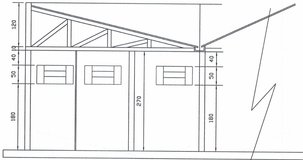
CORTE "AB"
