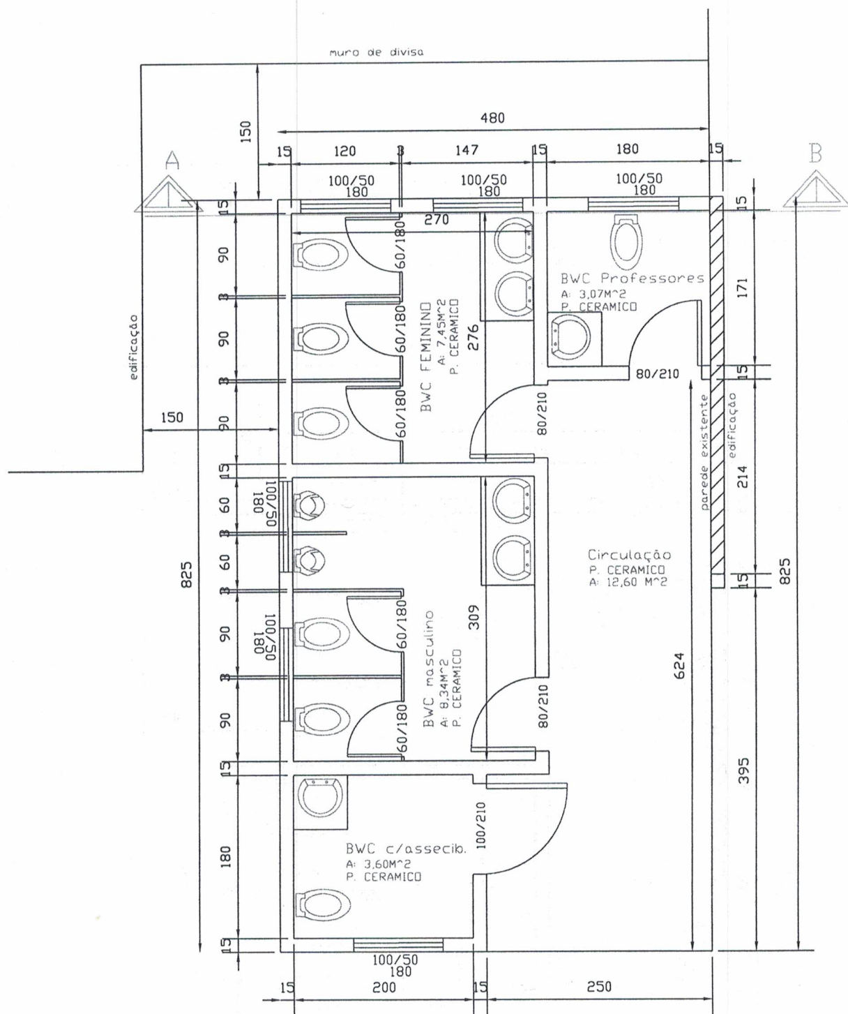
PLANTA BAIXA A= 39,60 m 2
