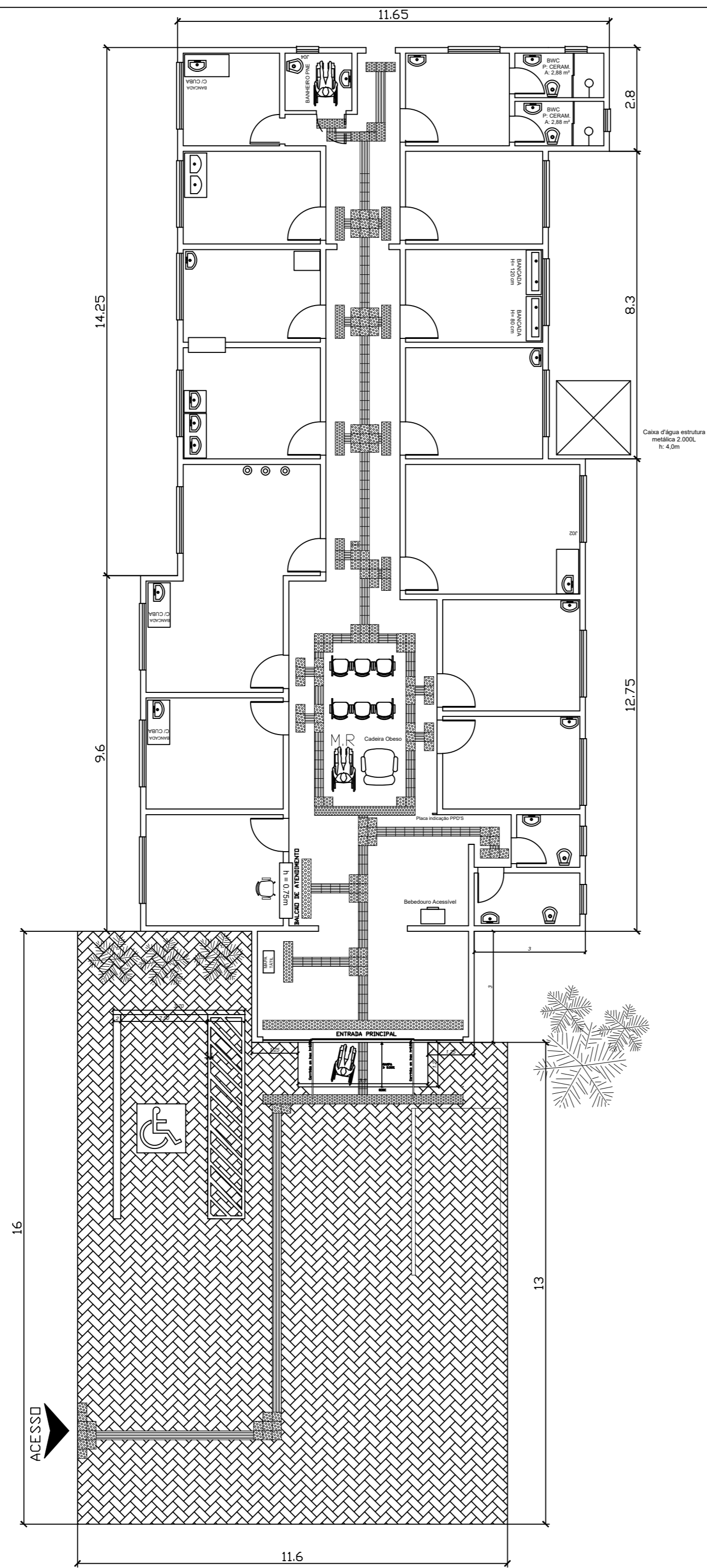
PLANTA BAIXA ESF I
