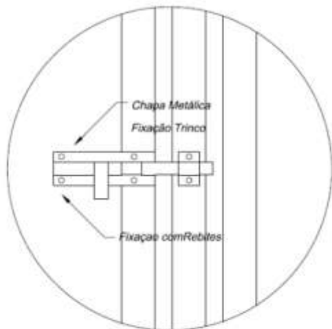
Detalhe Trinco Galvanizado
