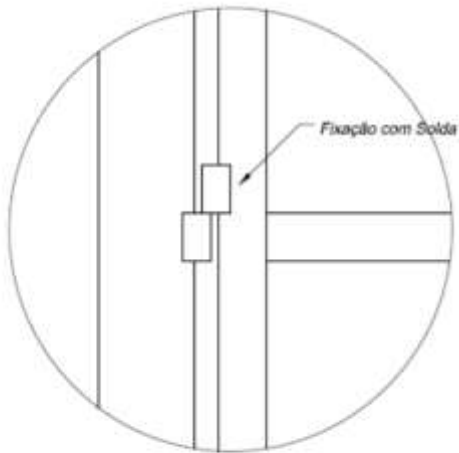
Detalhe Pino Gonzo 5/8
